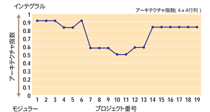
図15 アーキテクチャ指数の時系列変化
