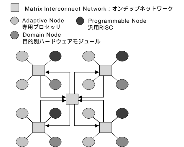
図5 Quicksilver ACMの構成
