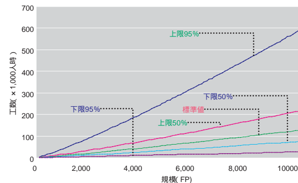
図3 規模あたりの工数の予測曲線と信頼幅
