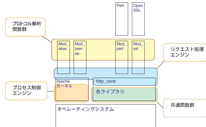
図10 Apache1.3.0の構造図とイメージ行列の関係
