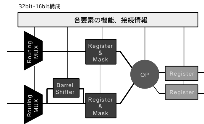
図4 動的リコンフィギュラブルプロセッサの構成要素の例 (Chameleon CS2112)
