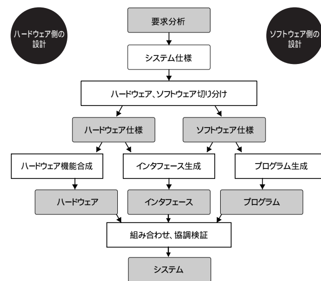
図2 協調設計の流れ
