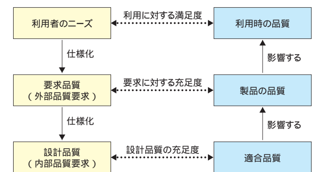
図2 ソフトウェア品質の概念とライフサイクルとの関係 (JIS X 0129-1:2003を元に、著者が修正した上で掲載)
