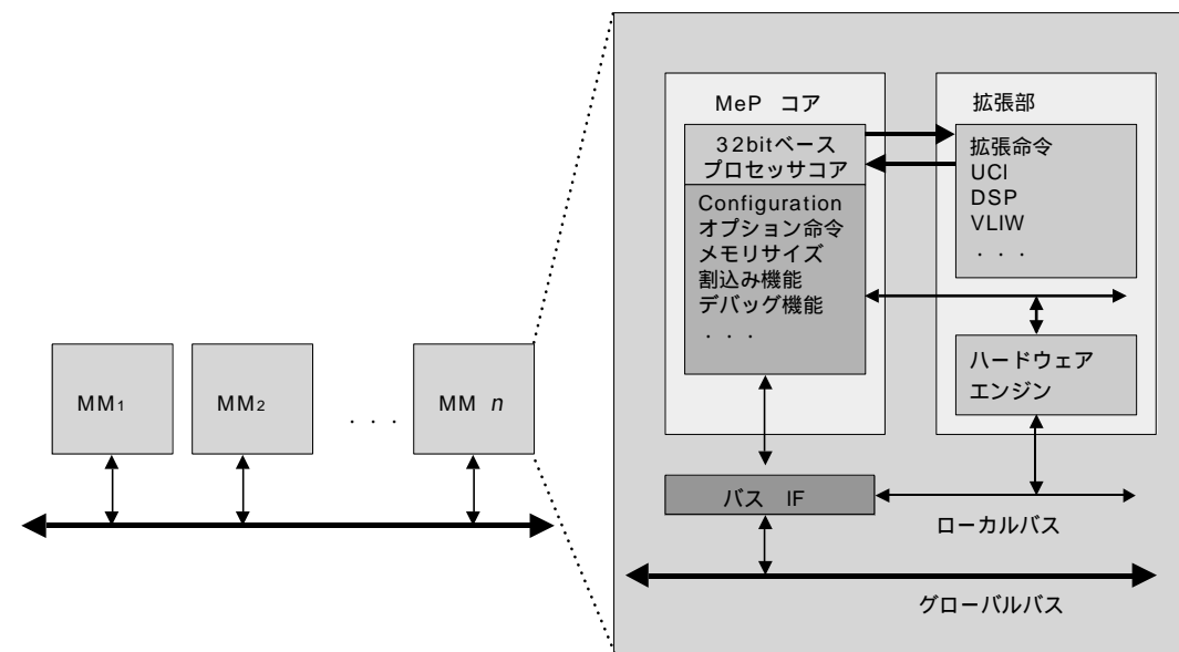
図6 東芝MePの構成
