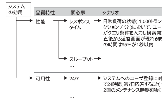
図3 ユーティリティ・ツリー例
