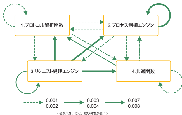
図11 縮約して得られたApache1.3.0のコールグラフ
