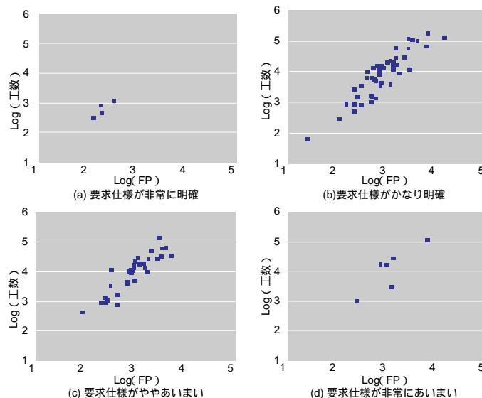
図4 「要求仕様の明確さ」に関するレベルごとの規模と工数の散布図
