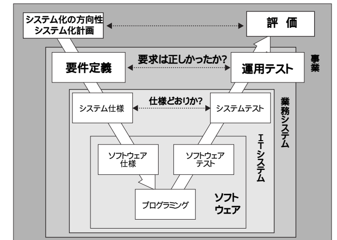
図1 要件定義・仕様とテストの関係
