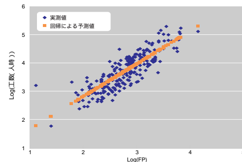
図2 規模と工数の散布図と回帰直線
