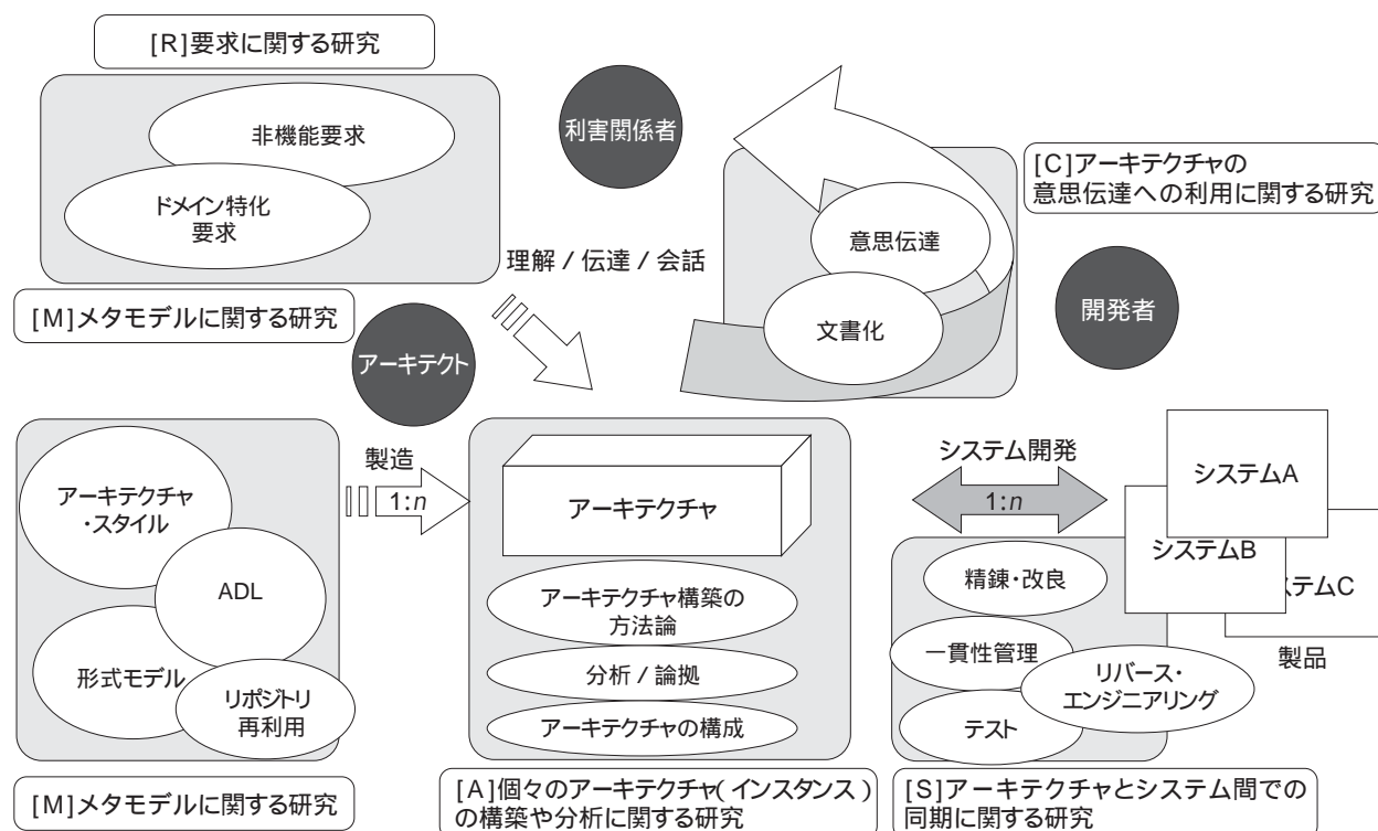
図2 ソフトウェア・アーキテクチャの果たす役割に注目し研究テーマを分類 文献[4]より
