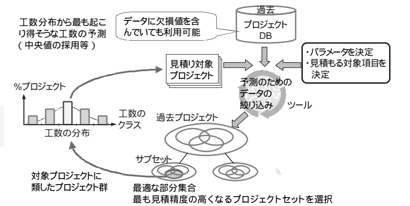
図4 OSR法による見積り手順
