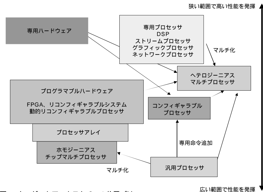
図7 ターゲットアーキテクチャの位置づけ
