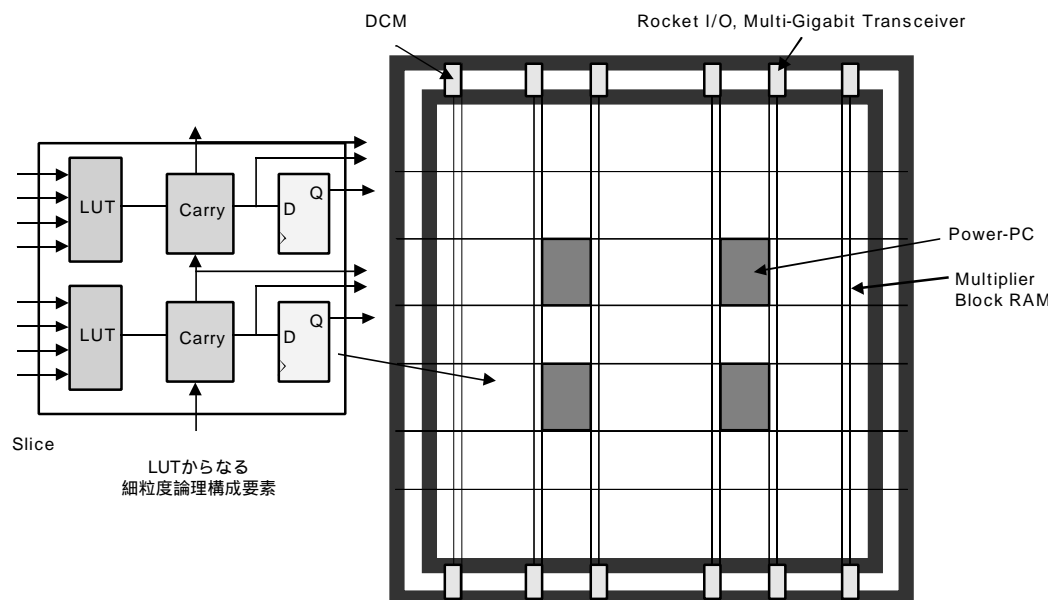
図3 組込みCPUとFPGAの混載例(Xilinx Virtex II Pro)
