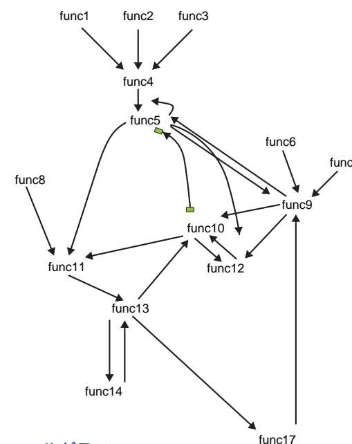
図7 コールグラフ
