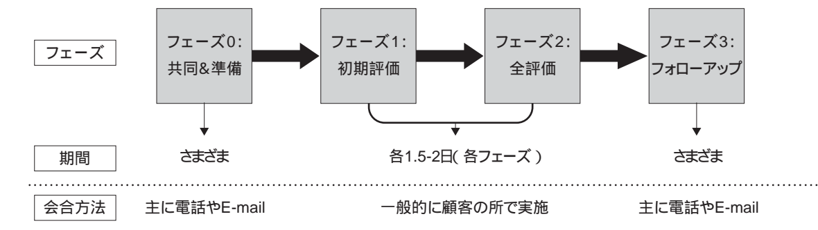
図4 ATAMの4フェーズ
